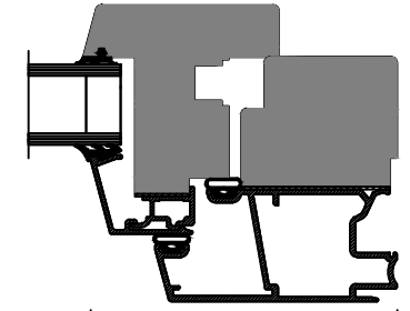
Jamb DK011
