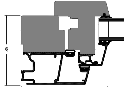
Jamb DK011
