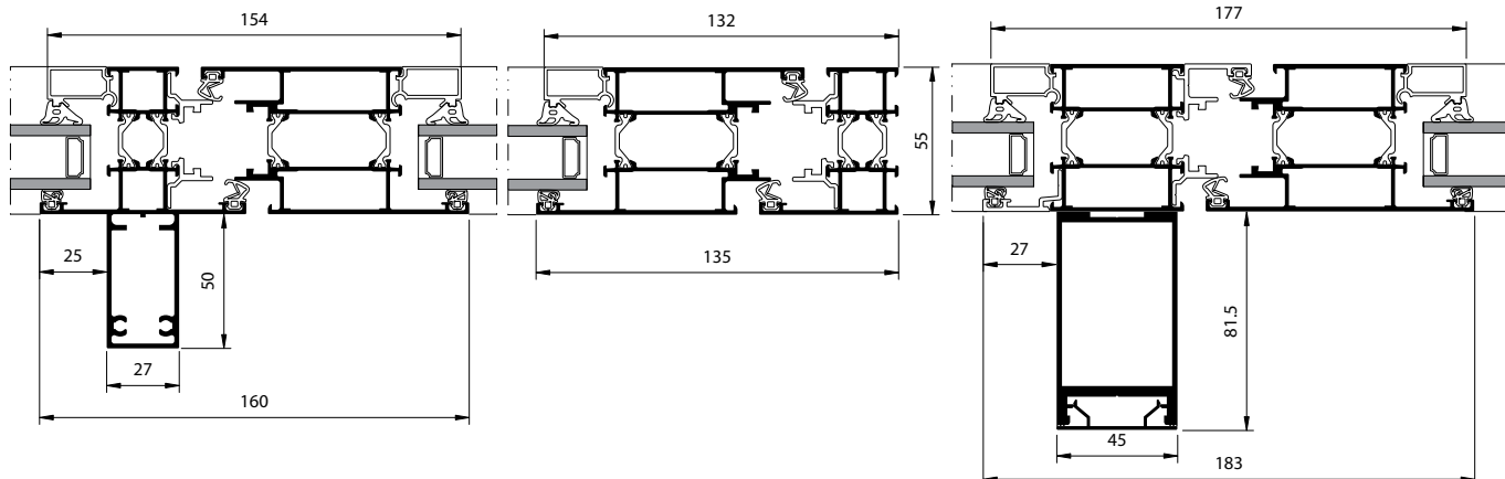
Coupe horizontale 1C - C' Horizontal cross section Corte horizontal
