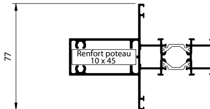
Meneau traverse Mullion - transom Montante - travesaño
