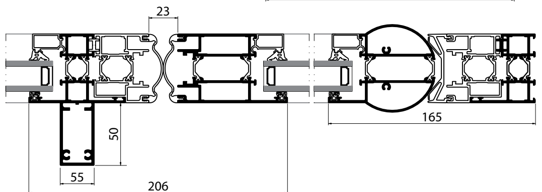
Coupe horizontale 1C - C'' Horizontal cross section Corte horizontal
