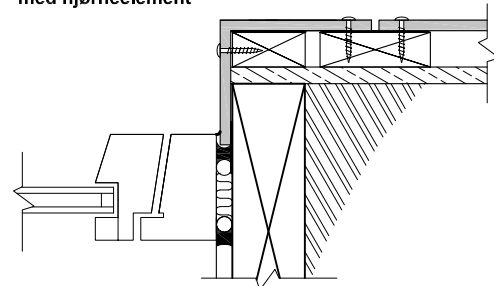
Horizontalsnitt Eksempel på vindusløsning med hjørneelement
