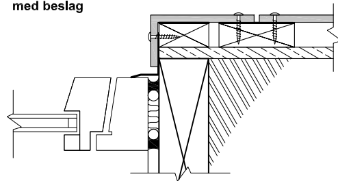
Horizontalsnitt Eksempel på vindusløsning med hjørneelement, kombinert med beslag
