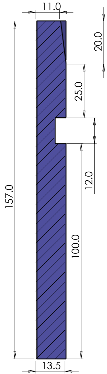
SECTION A-A SCALE 1 : 1
