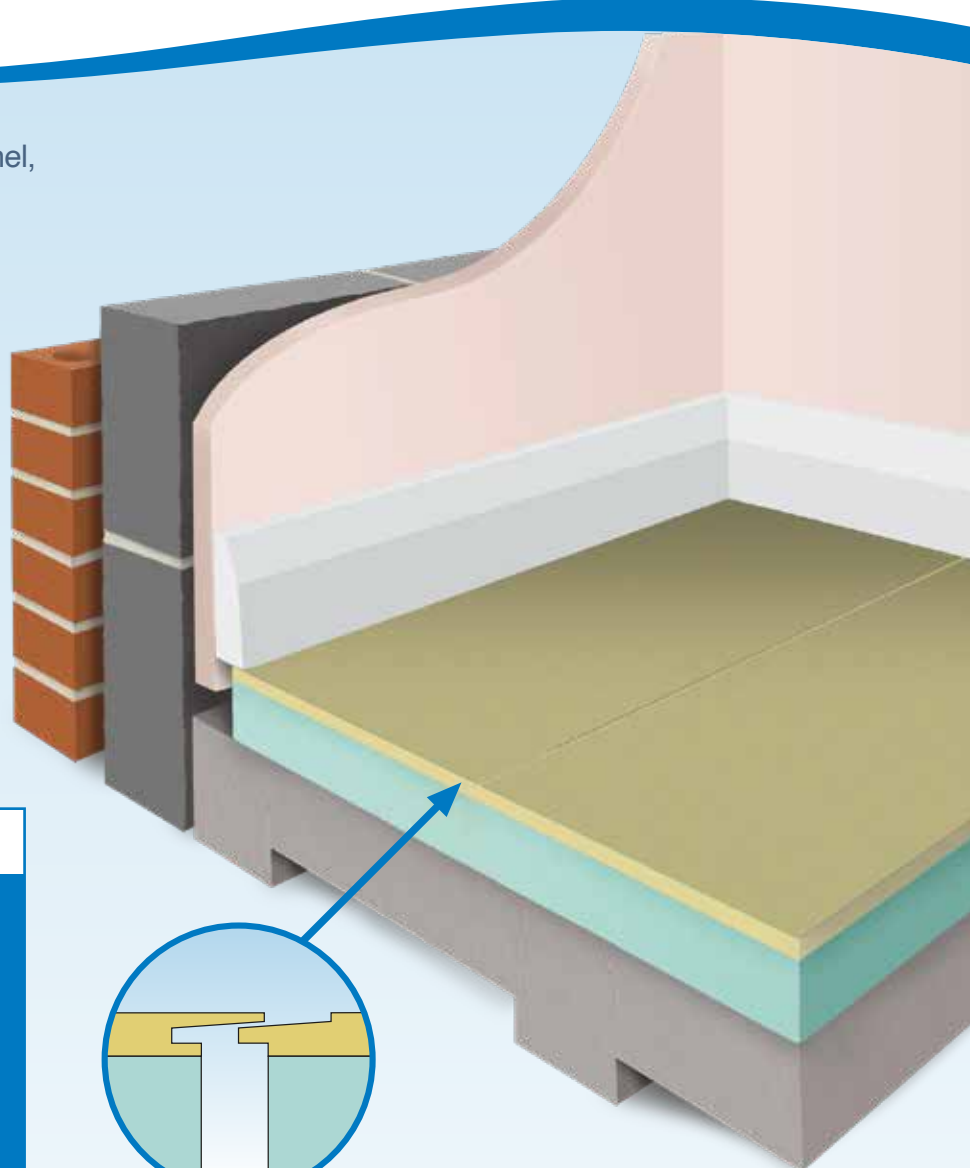
Tongue & Groove
