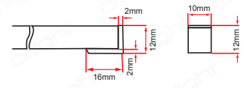
End Cap
