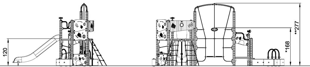
ELE400048BL ELE400048GR ELE400048RE 1:100
