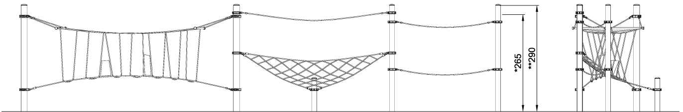
COR102401 1:100
