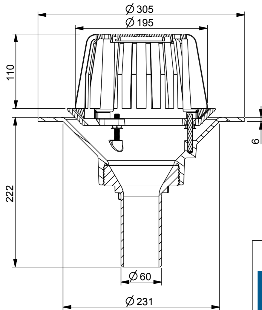
SECTION A-A
