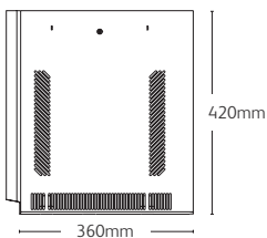
SL8 Tile Vent
