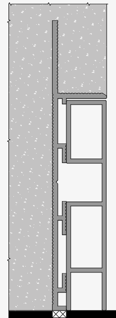
Flush baseboard with LED Plinthe affleurante avec LED
