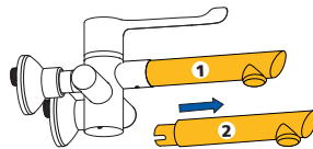
DELABIE ref.: H9610 - Principe de démontage
