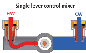
DELABIE ref.: H9610 coupe
