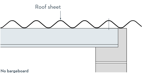
No bargeboard
