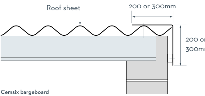
Cemsix bargeboard
