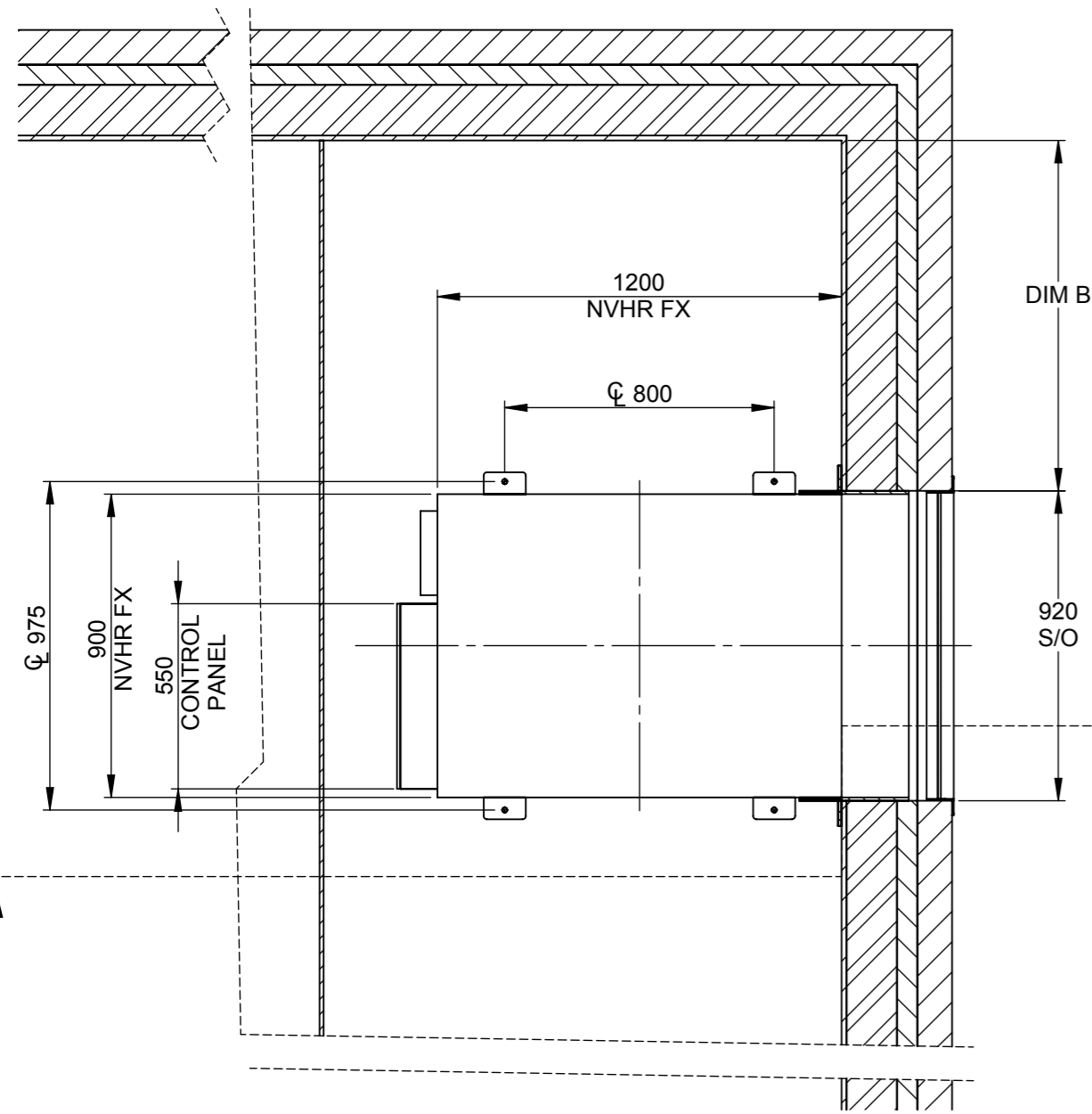
SECTION A-A
