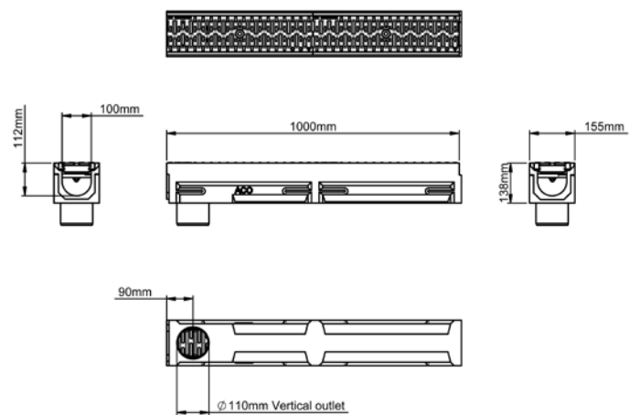
ACO Derailment Outlet Channel
