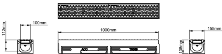
ACO Derailment Channel
